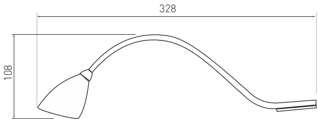
Rysunek techniczny produktu | Product technical drawing | Технический чертёж
