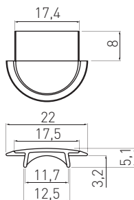
PA-ZASGLAX-00
