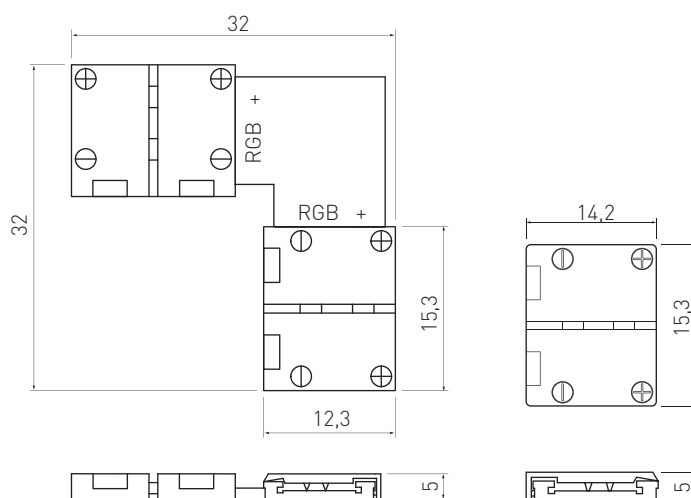
LD-ZTKTRGB-04N
