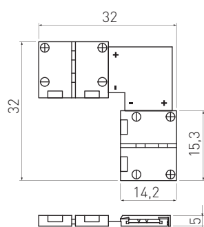
LD-ZTKT10MM-02N
