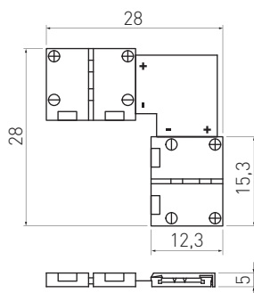
LD-ZTKT8MM-02N
